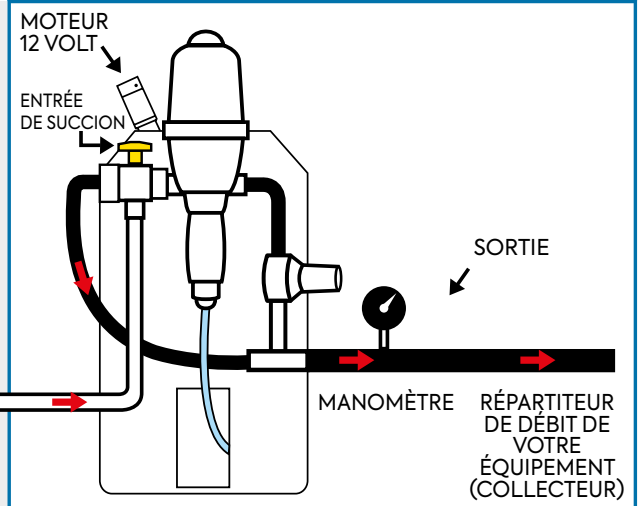
SYSTÈME D'INJECTION LIQUIDE AGTIV®
