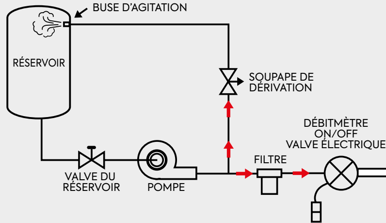
SYSTÈME EXISTANT D'APPLICATION DANS LE SILLON
